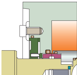
シングルメカニカルシール
