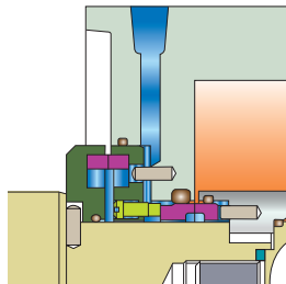
ダブルメカニカルシール
