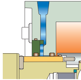
ダブル“O”リングシール
