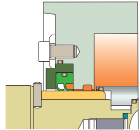
リップシール
