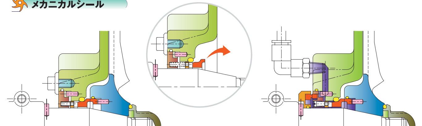
標準型メカニカルシール
